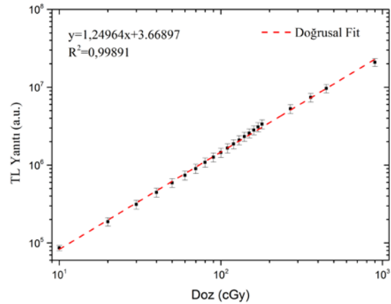
Şekil 9. Na 2 SO 4 örneklerine ait TL ışımaya eğrilerinin altında kalan alanlar kullanılarak elde edilen beta doz yanıt grafiği.
