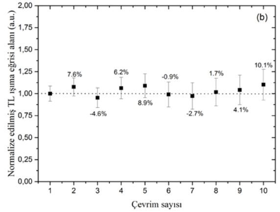
Şekil 10. \text{Na}_2\text{SO}_4 örneklerinden ışınlama-okuma çevrimi sonunda elde edilen a) TL ışıma eğrileri ve b) TL hassasiyetinin çevrim sayısı ile değişimi.
